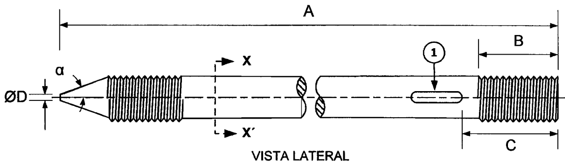
Figura 2: Jabalina de acero recubierta de cobre prolongable
