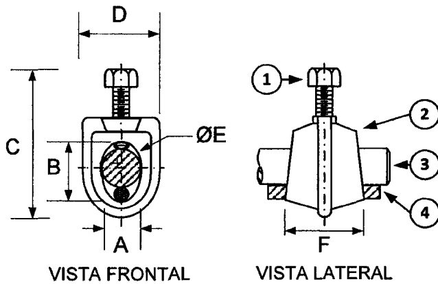
Figura 3: Conector tipo prensa
