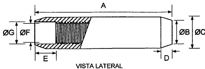
Figura 4: Conector tipo manguito
