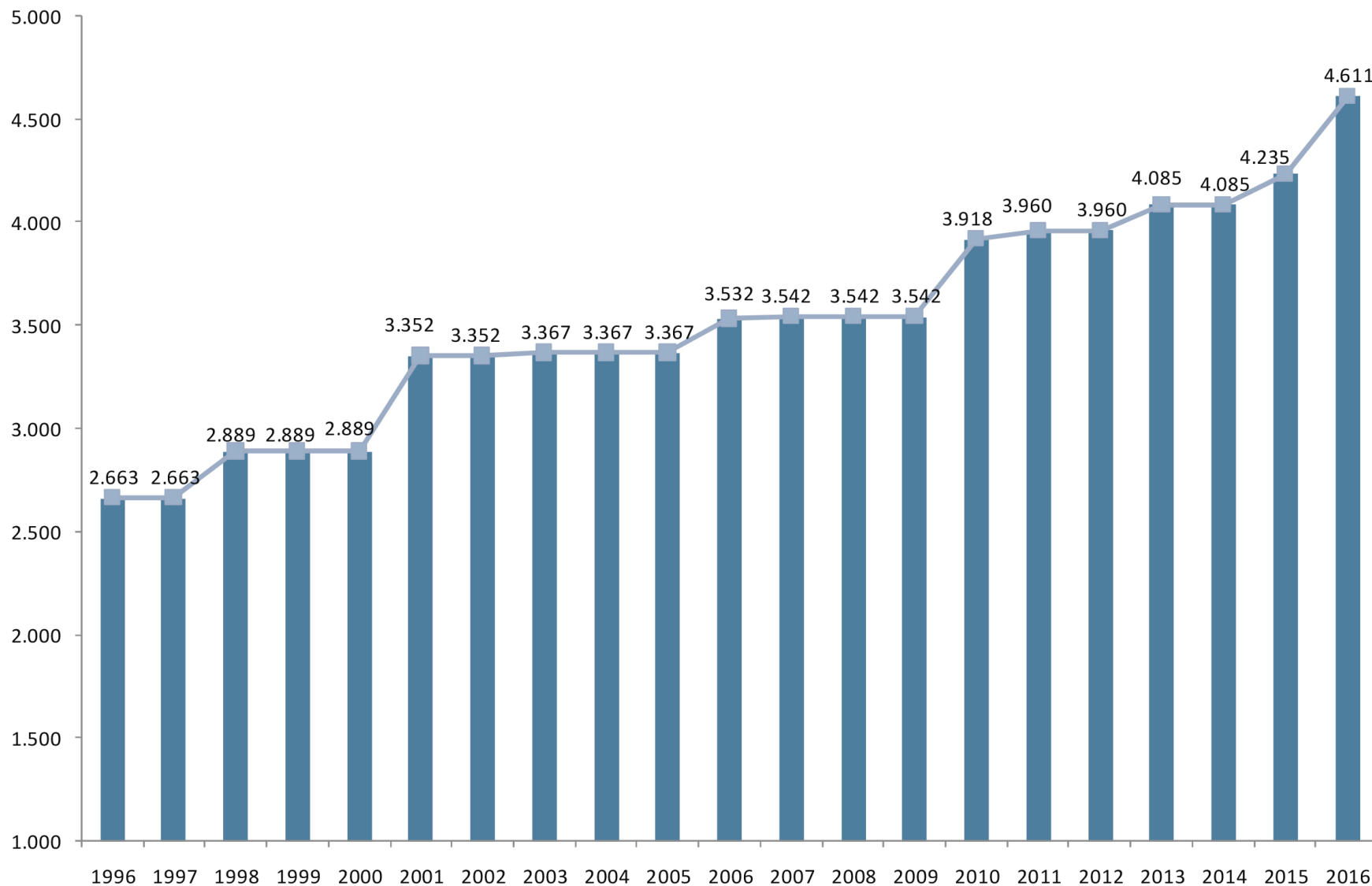
Longitud de Líneas de Transmisión en 220 kV, 1996-2016 (km)
