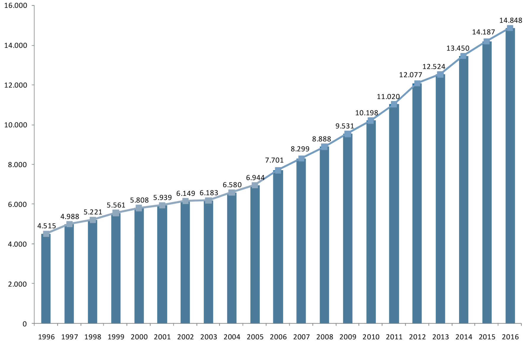
Consumo de Energía Eléctrica del SIN, 1996-2016 (GWh-Año)
