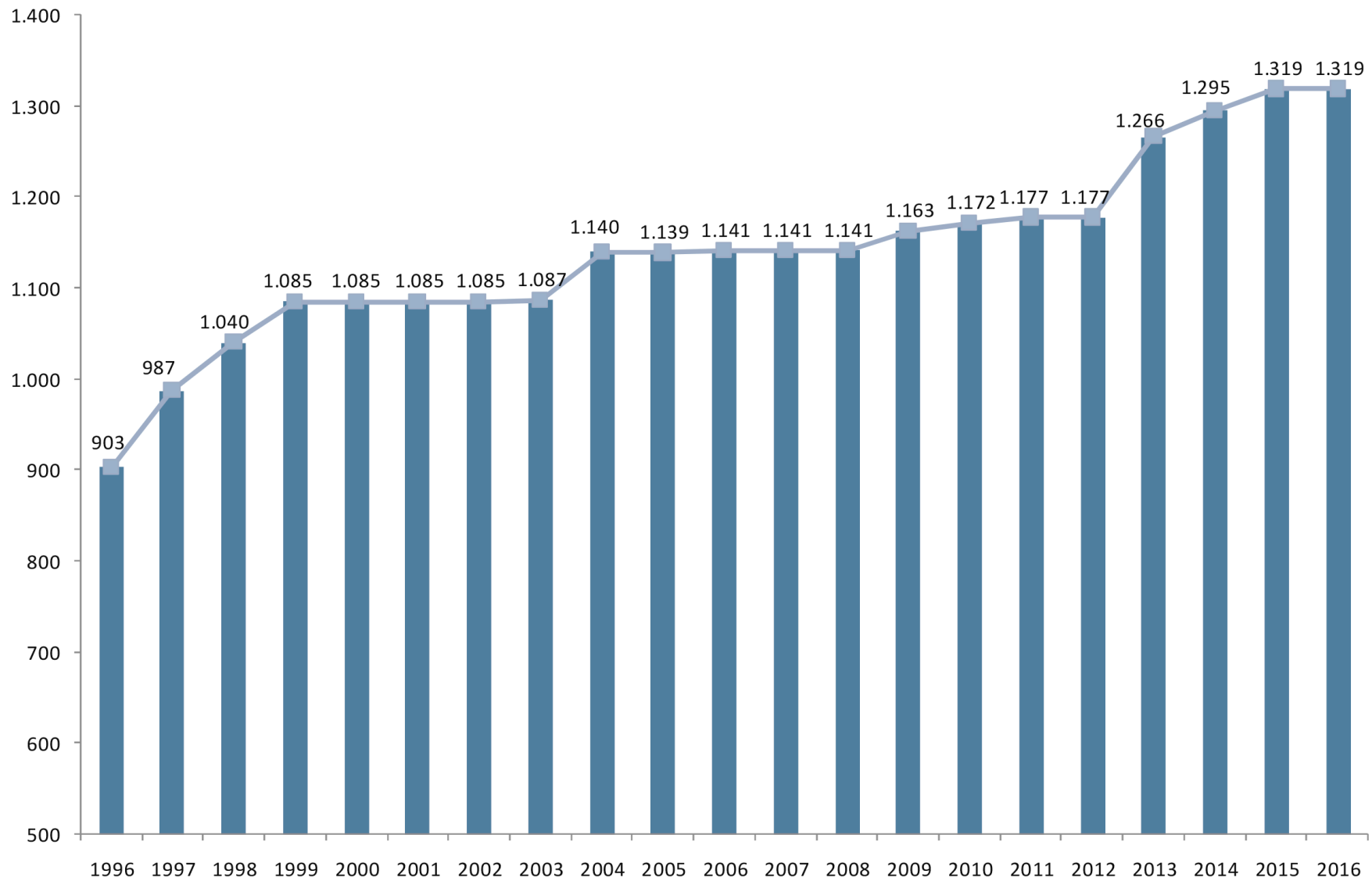
Longitud de Líneas de Transmisión en 66 kV, 1996-2016 (km)
