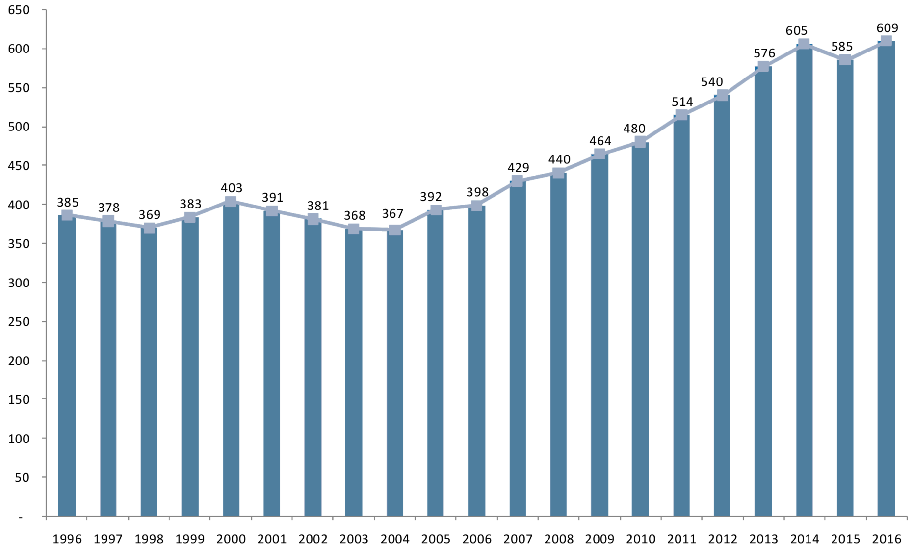
Consumo Total por Cliente - Mercado Nacional, 1996-2016 (kWh/Cliente-Mes)
