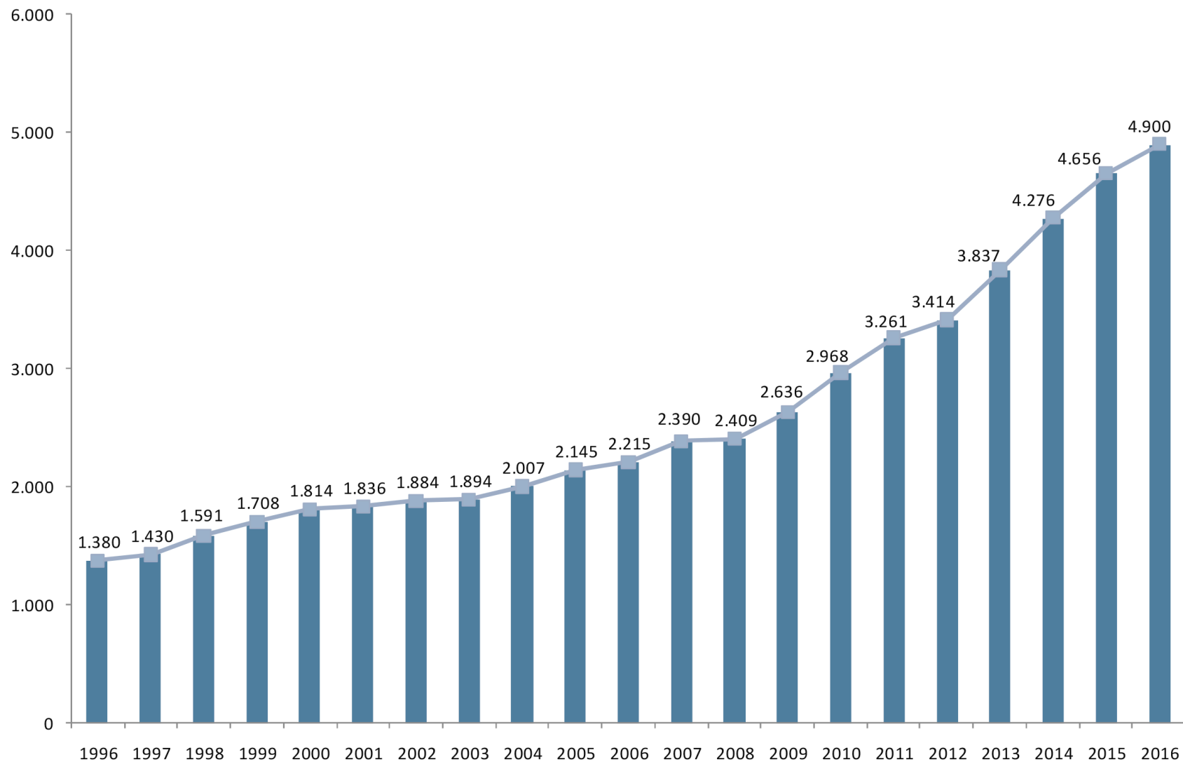
Potencia Instalada en 23 kV, 1996-2016 (MVA)
